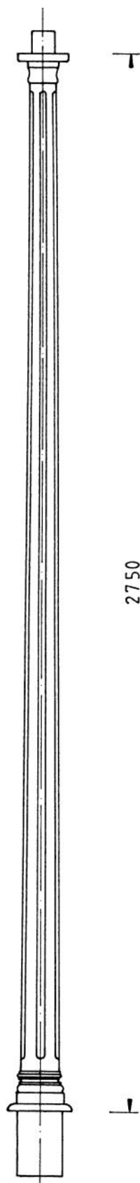
č. 635 L Stožár - část horní Dřík: 60mm Váha: 65 Kg
