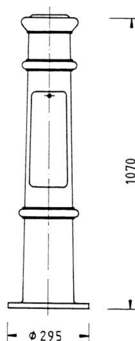
č. 635 A s dvířky Možno také bez dvířek Podstava stožáru - část spodní Instalace: patková (na základový prvek ) váha: 62Kg
