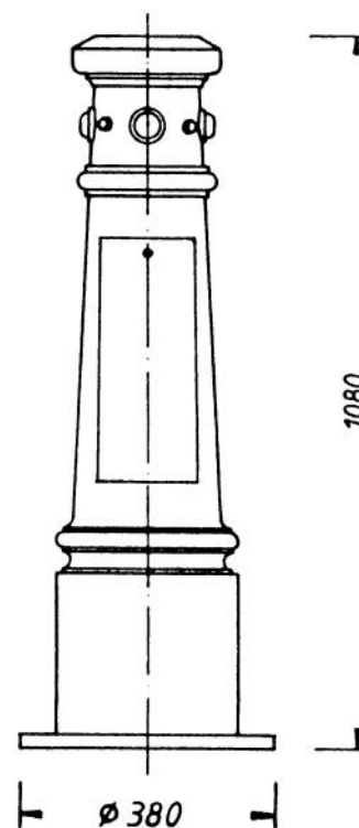
č. 640 A s dvířky Možno také bez dvířek Podstava stožáru - část spodní Instalace: patková (na základový prvek ) váha: 75Kg
