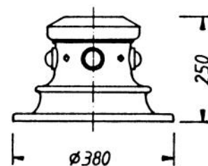
č. 640 C Krátká podstava stožáru Instalace: patková (na základový prvek ) váha: 30Kg
