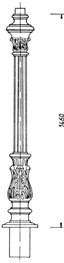
č. 640 K Stožár - část horní Dřík: 60mm Váha: cca 60 Kg
