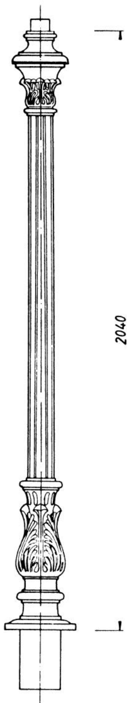
č. 640 Stožár - část horní Dřík: 60mm Váha: cca 80 Kg
