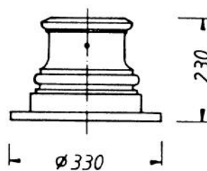
č. 655 C Krátká podstava stožáru Instalace: patková (na základový prvek ) váha: cca 29,5 Kg
