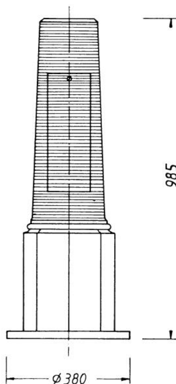
č. 660 A s dvířky Možno také bez dvířek Podstava stožáru - část spodní Instalace: patková (na základový prvek ) váha: cca 71 Kg
