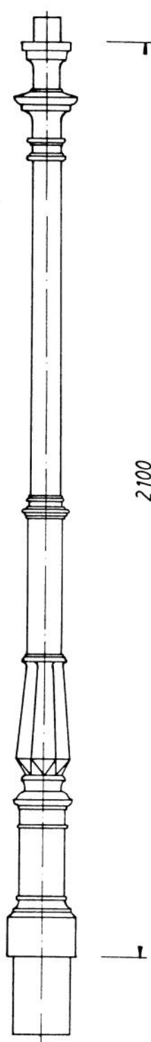
č. 660 Stožár - část horní Dřík: 60mm Váha: cca 55 Kg
