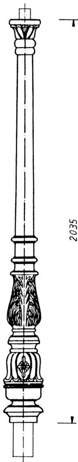
č. 690 Stožár - část horní Dřík: 60mm Váha: cca 95 Kg
