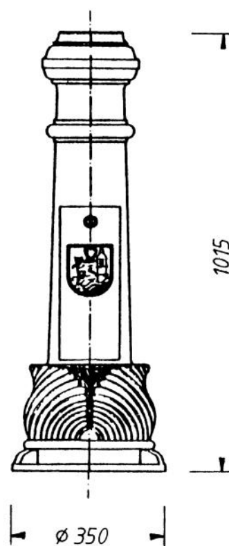
č. 690 A s dvířky Možno také bez dvířek Podstava stožáru - část spodní Instalace: patková (na základový prvek ) váha: cca 87 Kg
